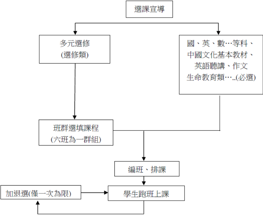
(一) 流程圖
